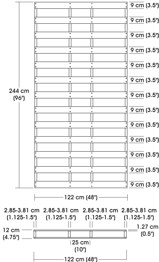
VISTA SUPERIOR
